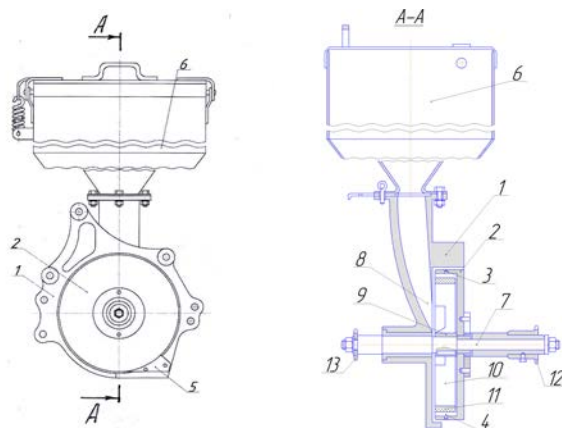
Рис. 1. Дозатор насіння сої з внутрішнім заповненням комірок висівного диска насінням: 1 – корпус; 2 – висівний диск; 3 – комірка; 4 – кільцева проточка; 5 – клиновий виштовхувач; 6 – насіннєвий бункер; 7 – вісь; 8 – вхідний отвір; 9 – крильчатка; 10 – лопаті; 11 – еластичні накладки; 12, 13 – приводні зірочки
