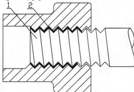
Рис. 2. Механізм стопоріння нарізного з'єднання за допомогою анаеробних матеріалів
