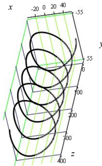
Рис. 4. Траєкторія руху виділеного об'єму вантажу у середньошвидкісному конвесрі: R=55 мм; \omega=15 рад/с
