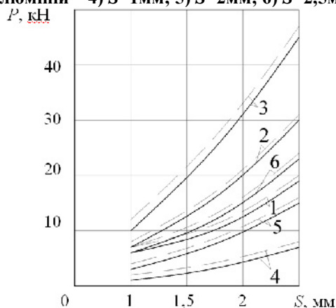
Рис. 3. Залежність сили гофроутворення від товщини стрічки ( t=40\text{мм} ; \alpha=80^\circ ): сталь 08кп – 1) b=20\text{мм} ; 2) b=40\text{мм} ; 3) b=60\text{мм} ; алюміній – 4) b=30\text{мм} ; 5) b=40\text{мм} ; 6) b=60\text{мм}
