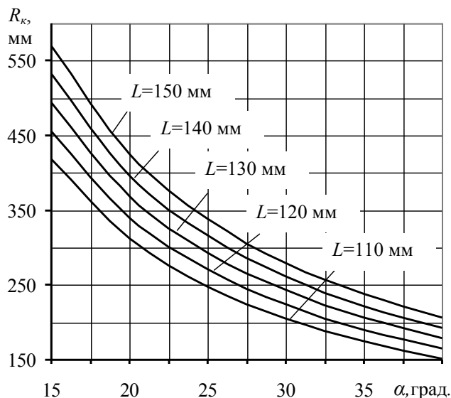
Рис. 5. Графічні залежності мінімального допустимого радіуса технологічної магістралі R_k від кута \alpha
